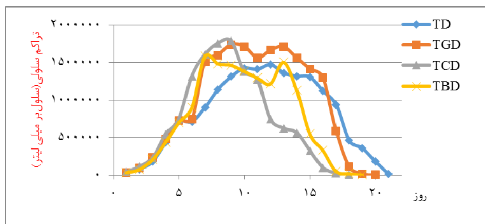
نمودار ۶: مقایسه منحنی رشد ریزجلبک Chlorella sp. در محیط کشت TMRL فاقد ویتامین و دارای ترکیبات ویتامین های مختلف در آب دریا
