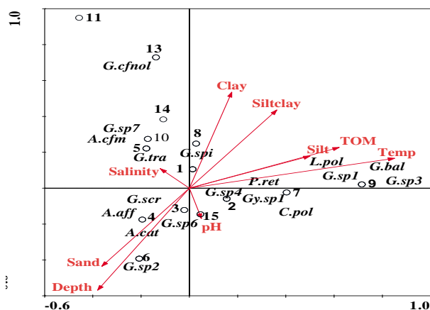
شکل ۳: نمودار سه پلاتی CCA در فصل بهار ۱۳۹۴، که جایگاه گونه‌ها، ایستگاه‌های نمونه برداری (نماد دایره) و پارامترهای محیطی (برداری) را در طول محور رسته‌بندی نشان می‌دهد. قرار گرفتن نام گونه در کنار نماد ایستگاه، نشان‌دهنده حضور گونه در آن ایستگاه است.
