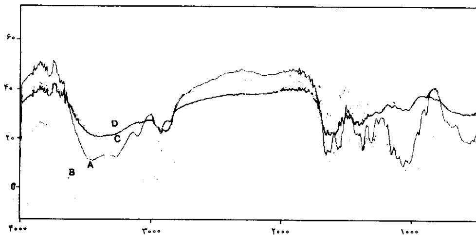
نمودار ۳: طیف FTIR مقایسه‌ای سه نوع کیتین با طیف نوع استاندارد A- طیف کیتین استخراجی از پوسته سیست آرتمیایورمیانا B- طیف کیتین استخراجی از پوسته میگو C- طیف کیتین استخراجی از پوسته خرچنگ D- طیف استاندارد کیتین (Sigma, 1999)
