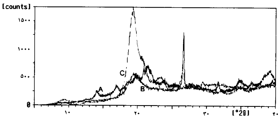
نمودار ۴: طیف‌های X-Ray مقایسه‌ای کیتین‌ها انجام شده با دستگاه X-Ray A- طیف مربوط به کیتین آرتمیایورمیانا (قرمز رنگ) B- طیف مربوط به کیتین پوسته خرچنگ (آبی رنگ) C- طیف مربوط به کیتین پوسته میگو (سبز رنگ) مشابهت ساختارهای بلوری حاصله بیانگر یکسان بودن مواد می‌باشد و اختلافات جزئی مربوط به منبع استخراجی و روش‌های عمل‌آوری و درصد رطوبت است.
