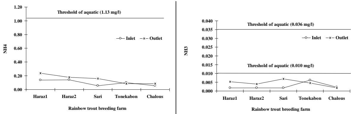
شکل ۹: تغییرات میانگین غلظت آمونیم و گاز آمونیاک در ایستگاه‌های ورودی و خروجی به همراه حد مجاز استاندارد کارگاه‌های پرورش ماهی قزل آلا منتخب استان مازندران (۱۴۰۰-۱۴۰۱)
