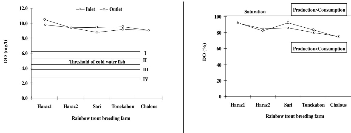
شکل ۴: تغییرات میانگین اکسیژن محلول و درصد اشباعیت اکسیژن در ایستگاه‌های ورودی و خروجی به همراه حد مجاز استاندارد کارگاه‌های پرورش ماهی قزل آلا منتخب استان مازندران (۱۴۰۰-۱۴۰۱)
