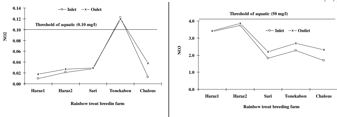
شکل ۱۰: تغییرات میانگین غلظت نیتريت در ایستگاه‌های ورودی و خروجی به همراه حد مجاز استاندارد کارگاه‌های پرورش ماهی قزل آلا منتخب استان مازندران (۱۴۰۰-۱۴۰۱)
