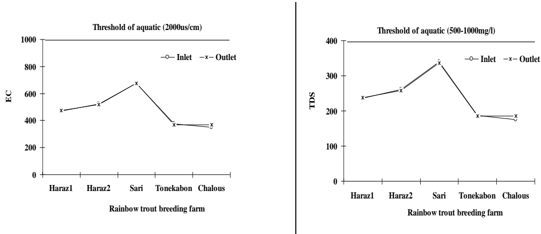
شکل ۶: تغییرات میانگین هدایت الکتریکی در ایستگاه‌های ورودی و خروجی به همراه حد مجاز استاندارد کارگاه‌های پرورش ماهی قزل آلا منتخب استان مازندران (۱۴۰۱-۱۴۰۰)
