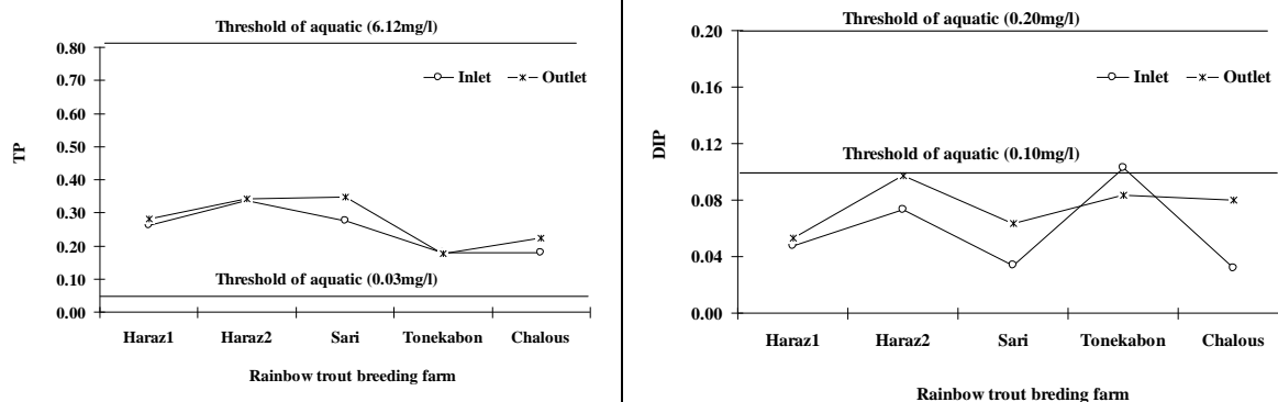
شکل ۸: تغییرات میانگین فسفر کل و فسفر معدنی در ایستگاه‌های ورودی و خروجی به همراه حد مجاز استاندارد کارگاه‌های پرورش ماهی قزل آلا منتخب استان مازندران (سال ۱۴۰۱-۱۴۰۰)
