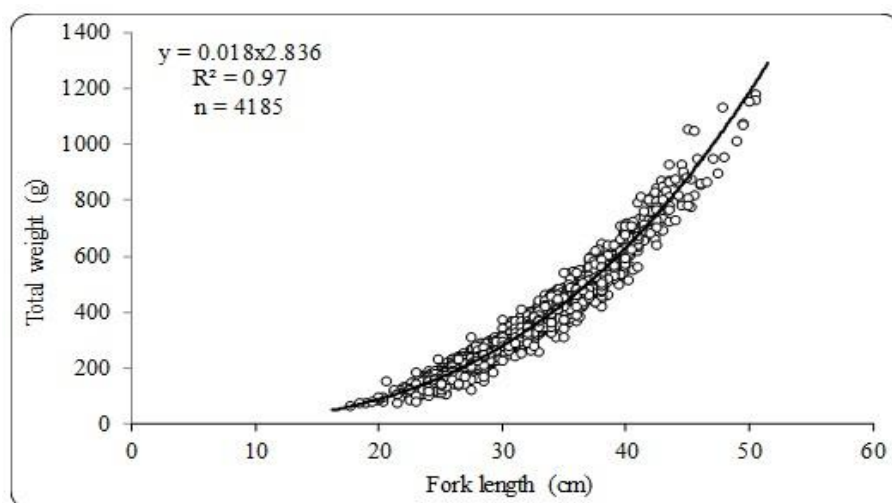
شکل ۲: رابطه طول چنگالی - وزن کل ماهی کفال طلایی طی سال‌های بهره‌برداری ۱۴۰۱-۱۴۰۲
