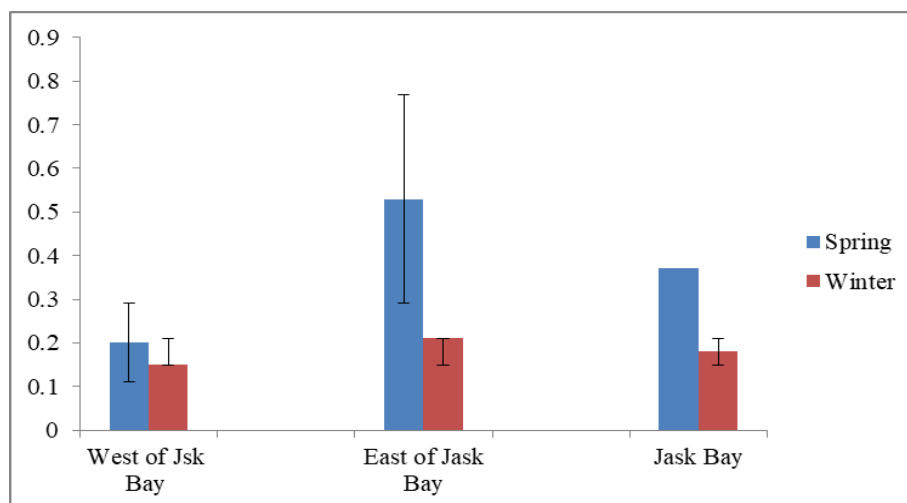
شکل ۲: تغییرات غلظت TPHs (میکروگرم بر کیلوگرم وزن خشک) رسوبات خلیج جاسک Figure 2: Concentration changes of TPHs ( \mu\text{g/kg} dry weight) in Jask Bay sediments
