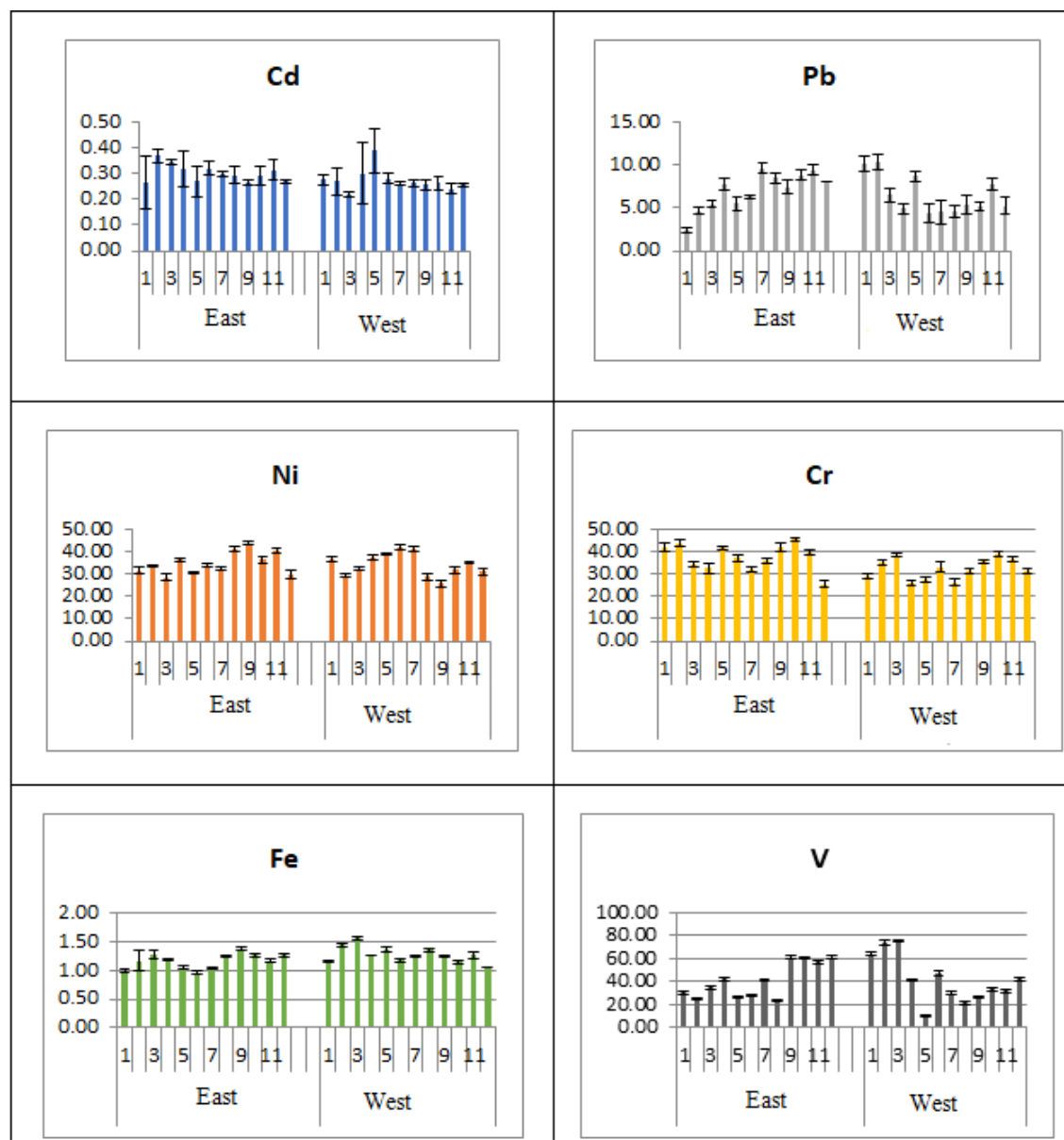
شکل ۴: تغییرات غلظت (میکروگرم بر گرم وزن خشک) فلزات سنگین در رسوبات خلیج جاسک (زمستان ۱۴۰۲) Figure 4: Concentration changes of heavy metals ( \mu\text{g/kg} dry weight) in Jask Bay sediments (winter, 1402)
