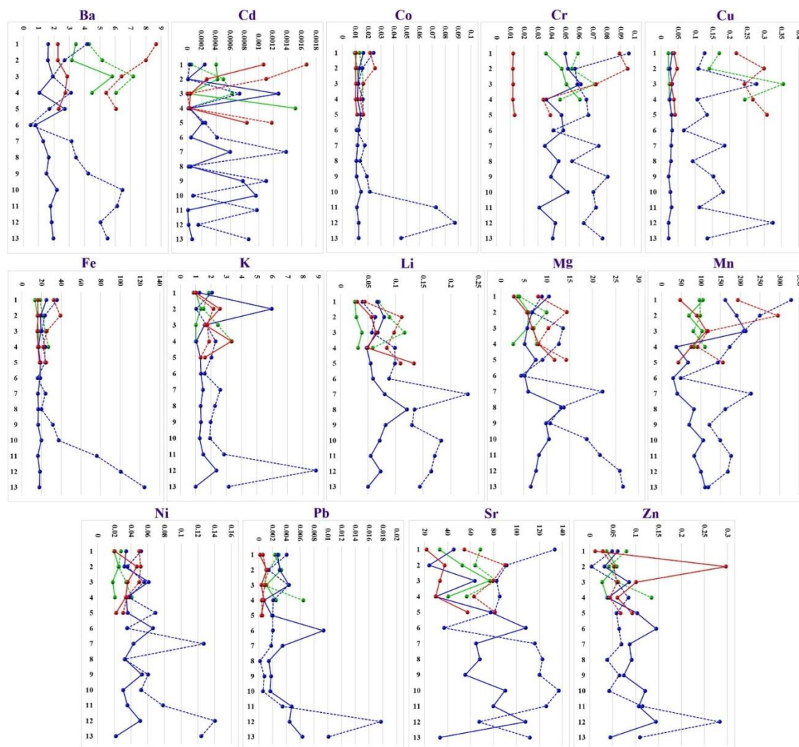
شکل ۷: نسبت های عناصر به کلسیم اندازه گیری شده در نقاط انتخابی در لایه های پریماتیک (خطوط نقطه چین) و نکرئوس (خطوط ممتد) در مقاطع عرضی پوسته صدف نمونه های Anodonta anatina گردآوری شده از سه ایستگاه نمونه برداری (ایستگاه های ۱، ۲ و ۳ به ترتیب با رنگ های قرمز، آبی و سبز نشان داده شده اند). محور عمودی نشان دهنده نقاط تجزیه و تحلیل متوالی از ناحیه آمو تا حاشیه شکمی است (اعداد نشان دهنده سن لایه های مربوطه بر حسب سال است). محور افقی نسبت های اندازه گیری شده (عنصر به کلسیم) را بر حسب میلی مول بر مول نشان می دهد.
