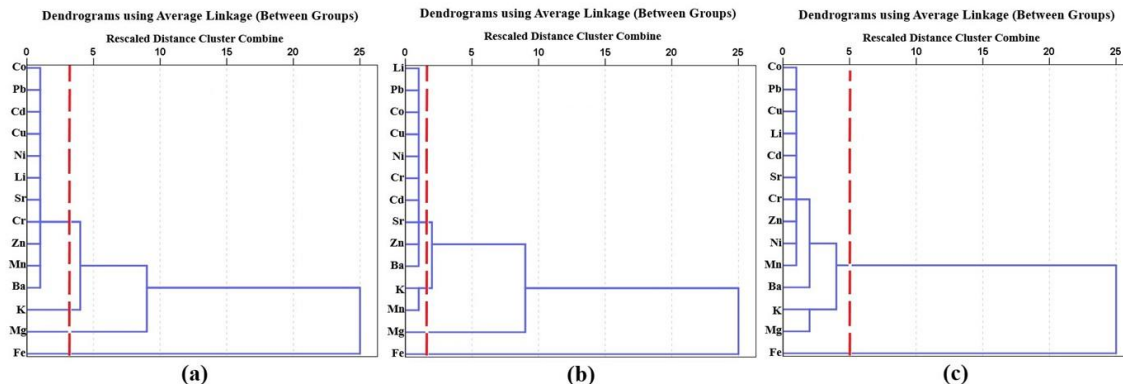
شکل ۴: طبقه‌بندی عناصر انتخابی در رسوبات مغزه‌ای گردآوری شده از ایستگاه‌های نمونه‌برداری (a, b و c: به ترتیب ایستگاه‌های ۱ الی ۳) که بر اساس تجزیه و تحلیل خوشه‌ای سلسله مراتبی (HCA) با به کارگیری روش پیوند میانگین، با فواصل اقلیدسی حاصل شده است. خط‌چین‌های عمودی نشانگر گروه‌بندی خوشه‌هاست.
