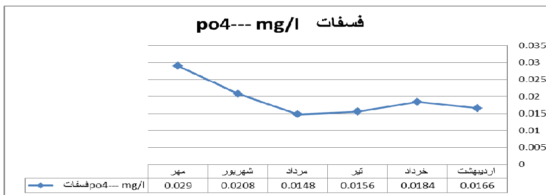
شکل ۱۰: فسفات ( \text{PO}_4^{3-} ) آب کانال محمدیه، محدوده استان تهران
