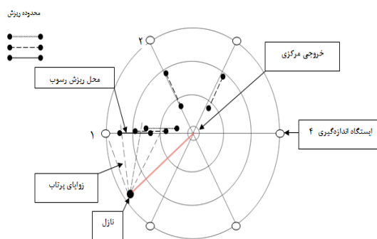
شکل ۲: موقعیت پرتاب جت آب در مخزن Figure 2: Outlet orientation in the tank
