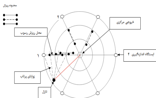
شکل ۲: موقعیت پرتاب جت آب در مخزن
