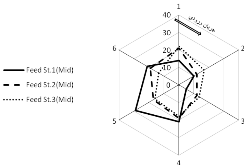
شکل ۵: الگوی کمی رسوب گذاری با ریزش رسوب در قسمت بینابینی شعاع مخزن در ایستگاه های ۱، ۲ و ۳
