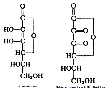
شکل ۱: فرمول گستره شیمیایی ال-آسکوربیک اسید (چپ) و دهیدرو-ال-آسکوربیک اسید (فرم اکسید شده) (راست) Figure 1: Chemical Formula of L-Ascorbic acid (left) and Dehydro L-Ascirbic acid (Right)
