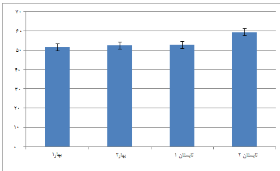
شکل ۳: میانگین شاخص کیفیت آب در مراحل مختلف نمونه برداری Figure 3: Average water quality index in different stages of sampling
