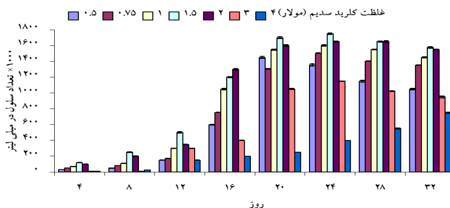
شکل ۴: میانگین \pm انحراف معیار تعداد سلول‌های جلبک Dunaliella sp. در غلظت‌های مختلف کلرید سدیم طی روزهای مختلف کشت
