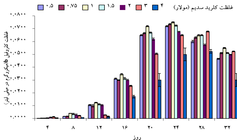
شکل ۶: میانگین \pm انحراف غلظت کلروفیل b جلبک Dunaliella sp. در غلظت‌های مختلف کلرید سدیم طی روزهای مختلف کشت
