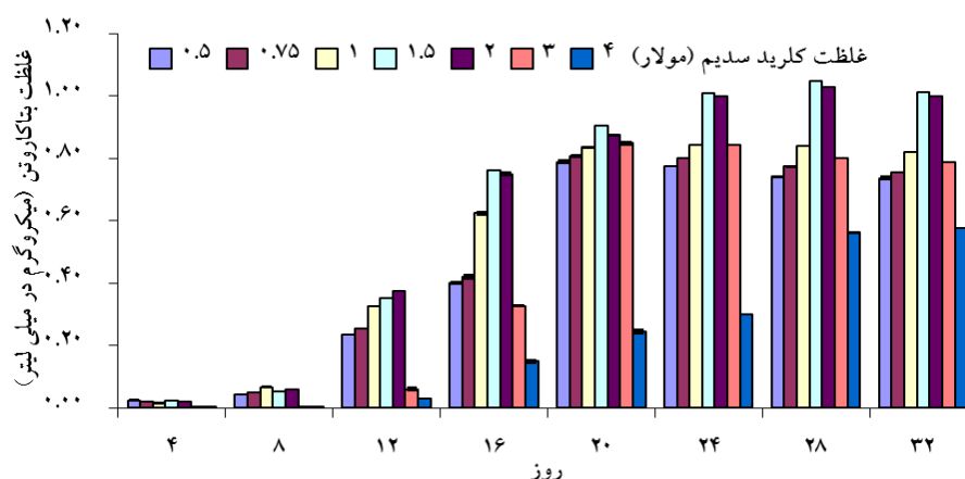
شکل ۷: میانگین \pm انحراف غلظت بتاکاروتن جلبک Dunaliella sp. در غلظت‌های مختلف کلرید سدیم طی روزهای مختلف کشت Figure 7: The mean \pm SD density of Dunaliella sp. isolated \beta -carotene in different levels of NaCl during different days.
