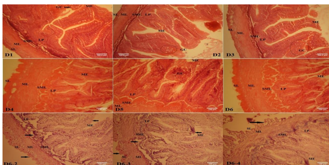
شکل ۴- آسیب‌شناسی بافت روده ماهی‌ها در ایستگاه‌های مختلف؛ ایستگاه اول، دوم و ایستگاه سوم (شکل D1-D3)، و ایستگاه چهارم (شکل D4-D6). غشای سروزی (SL)، سلول‌های جامی (GC)، لایه عضلانی (ME)، اپیتلیوم مخاطی (ML)، لامینا پروپریا (LP) و لایه زیر مخاطی (SML)
