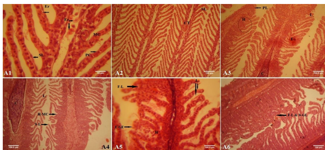
شکل ۱: آسیب‌شناسی بافت آبشش ماهی‌ها در ایستگاه‌های مختلف: ایستگاه اول و دوم (شکل A1 و A2)، ایستگاه سوم و چهارم (شکل A3-A6). ادم (E)، هیپرتروفی (H)، عروق آوران (AV)، گلبول قرمز (Er)، سلول‌های ستونی (PC)، سلول مخاطی (MC)، لاملاهای ثانویه (SL) و لاملاهای اولیه (PL)
