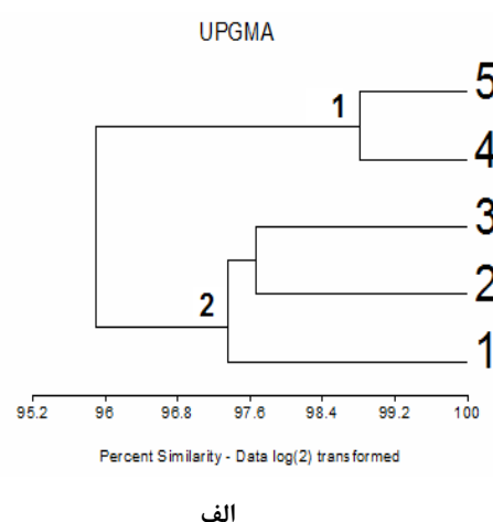
شکل ۳: آنالیز خوشه‌ای پارامترهای فیزیکو-شیمیایی آب در ایستگاه‌ها (الف) و ماه‌های (ب) مختلف دریاچه سد آزاد سنندج (سال های ۹۵-۱۳۹۴)
