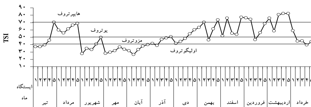
شکل ۲: تغییرات TSI کل در ایستگاهها و ماههای مختلف در دریاچه سد آزاد سنندج (سالهای ۹۵-۱۳۹۴)
