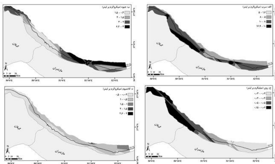
شکل ۳: روند تغییرات فلزات سنگین در محدوده خشت‌سر تا کياشهر در فصل‌های پاييز، زمستان و بهار Figure 3: The trend of heavy metals within Khesht Sar to Kiashahr in autumn, winter and spring.
