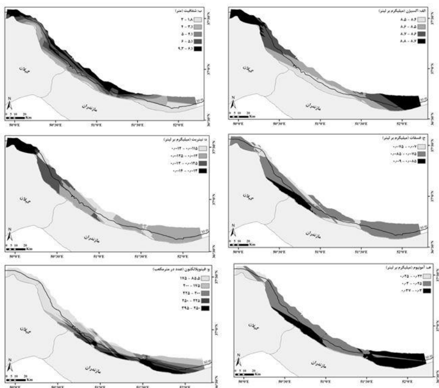
شکل ۲: روند تغییرات پارامترهای زیستی و غیرزیستی در محدوده خشت‌سر تا کياشهر در فصول پاييز، زمستان و بهار Figure 2: The trend of biotic and abiotic parameters within Khesht Sar to Kiashahr in autumn, winter and spring.
