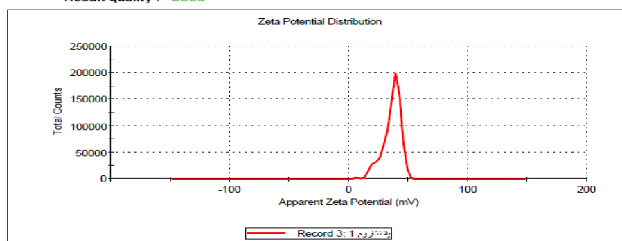
شکل ۴: پتانسیل زتای ریزپوشینه‌ها با استفاده از آلژینات (با ویسکوزیته متوسط) و کیتوزان (با وزن مولکولی پایین). pH محلول آلژینات و کیتوزان ۳/۵ بود.
