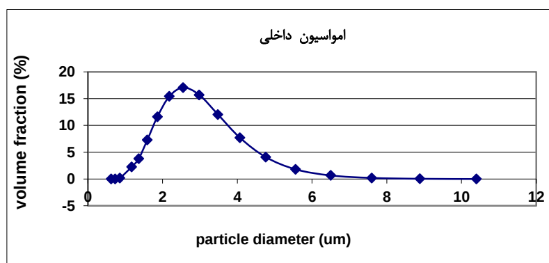
شکل ۳: نحوه پراکنش اندازه ذرات ریزپوشینه و درصد فراوانی آن‌ها بر اساس داده‌های دستگاه پارتیکل سایز آنالایزر Figure 3: Particle size distribution of microcapsules using ionic gelation and frequency are based on data Particle Size Analyzer.
