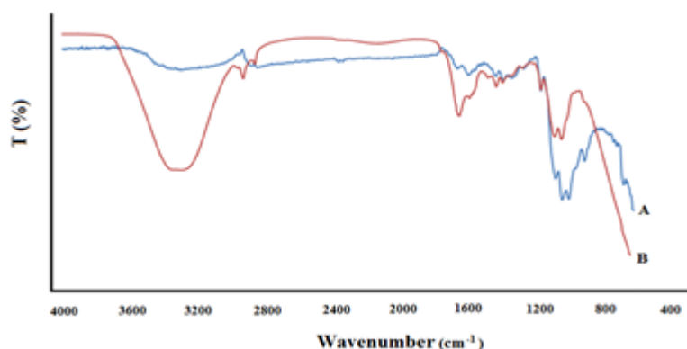
شکل ۴: طیف FTIR مربوط به کیتوزان خام و کمپوزیت کیتوزان حاوی اکسید نقره Figure 4: FTIR analysis of raw chitosan and AgO-chitosan composite
