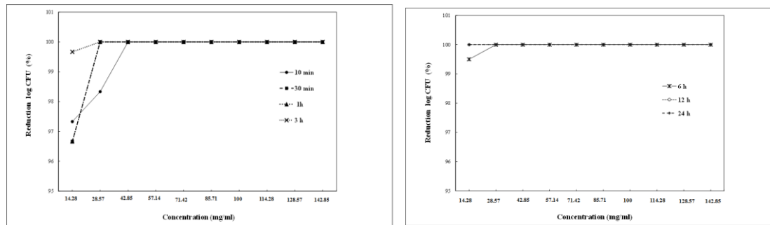
شکل ۷: نتایج حاصل از اثر بنتونیت اصلاح شده بر کاهش میزان باکتری یرسینیا راکری در تیمارهای مختلف Figure 7: Percent reduction in the number at different time and concentrations AgO-chitosan composite.
