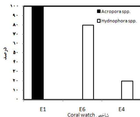
شکل ۵: درصد سلامت جوامع مرجانی جزیره هندورابی در تابستان ۱۳۹۶
