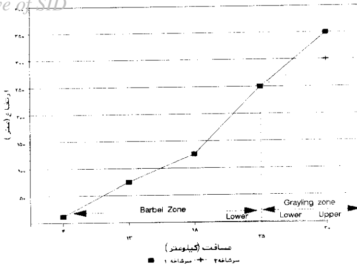
نمودار ۷: پروفیل طولی و ناحیه‌بندی رودخانه شمروند
