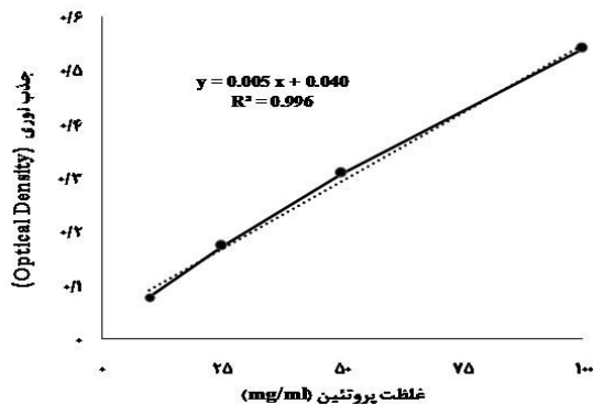
شکل ۱: منحنی استاندارد BSA (غلظت ۱ mg/ml). [محور X : غلظت پروتئین (mg/ml)؛ محور Y: جذب نوری] Figure 1: Standard curve of BSA (1 mg / ml) [X axis: protein concentration (mg/ml) ; Y axis: Optical Density]
