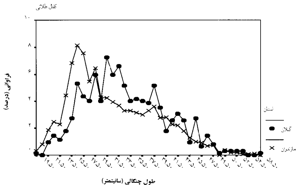
نمودار ۳: توزیع فراوانی طول چنگالی ماهی کفال طلایی در سال ۸۰-۱۳۷۹
