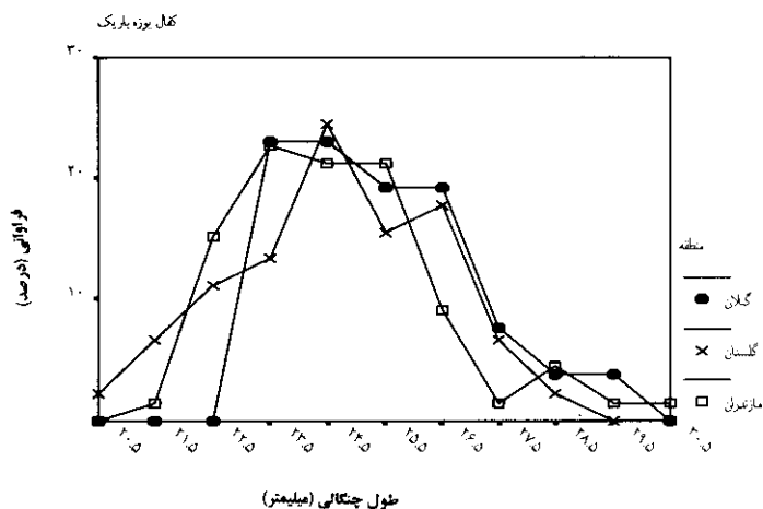
نمودار ۶: توزیع فراوانی طول چنگالی ماهی کفال پوزه باریک در سال ۸۱-۱۳۸۰
