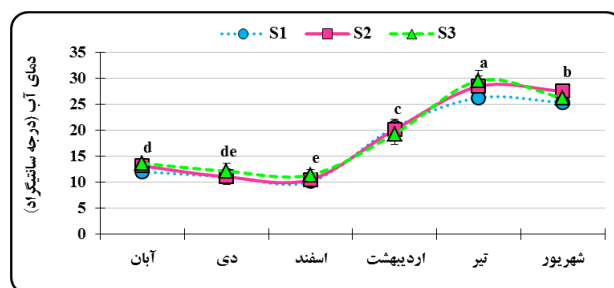
شکل ۲: مقایسه میانگین ( \pm انحراف معیار) دمای آب بر حسب ایستگاه‌ها و ماه‌های مختلف نمونه‌برداری در مصب چشمه کیله تنکابن. حروف نامتشابه بیانگر اختلاف معنی‌دار در بین میانگین‌ها است ( p < 0.05 ).
