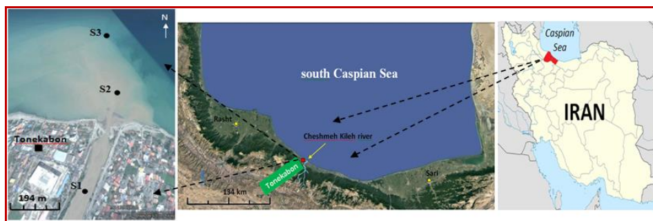
شکل ۱: موقعیت مکانی مصب چشمه کیله تنکابن و ایستگاه‌های مورد مطالعه (۹۴-۱۳۹۳)
