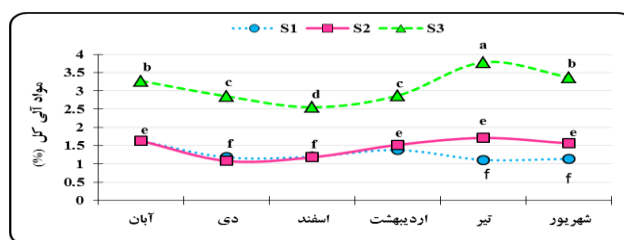
شکل ۴: مقایسه میانگین ( \pm انحراف معیار) درصد مواد آلی رسوبات بستر بر حسب ایستگاه‌ها و ماه‌های مختلف نمونه‌برداری در مصب چشمه کیله تنکابن. حروف نامتشابه بیانگر اختلاف معنی‌دار در بین میانگین‌ها است ( p < 0.05 ).
