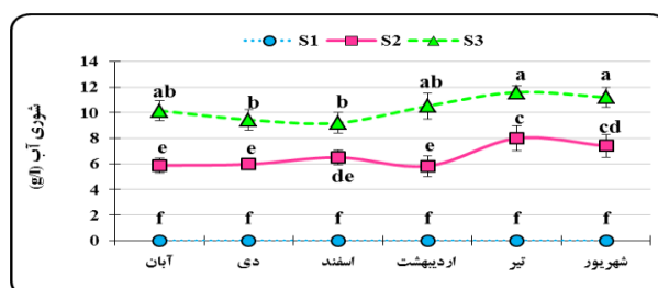
شکل ۳: مقایسه میانگین ( \pm انحراف معیار) شوری آب بر حسب ایستگاه‌ها و ماه‌های مختلف نمونه‌برداری در مصب چشمه کیله تنکابن. حروف نامتشابه بیانگر اختلاف معنی‌دار در بین میانگین‌ها است ( p < 0.05 ).
