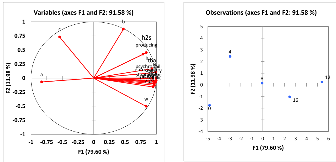
شکل ۲: تحلیل مولفه های اصلی (PCA) مطالعه پارامترهای کیفی ماهی کفال پشت سبز شکم خالی نگهداری شده در یخ: (a) پارامترها شاخص کیفی شامل: ویژگی های حسی، رنگ سنجی، باکتری مزوفیل، باکتری سرمادوست، باکتری انتروباکتریاسه، باکتری استافیلوکوکوس، باکتری تولید کننده H 2 S، بازهای ازته فرار، تری متیل آمین، pH، تیوباربتوریک اسید، اسیدهای چرب آزاد (b) = روز ۰، روز ۴، روز ۸، روز ۱۲، روز ۱۶ و روز ۱۶.
