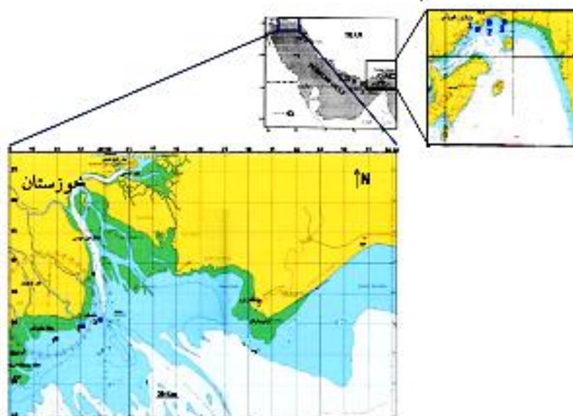
شکل ۱: نقشه منطقه نمونه برداری Figure 1: Location of the study area.
