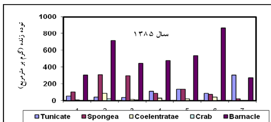
نمودار ۱۰-۳: میزان توده زیاده گروههای اصلی روی انواع سازه در سال ۱۳۸۵
