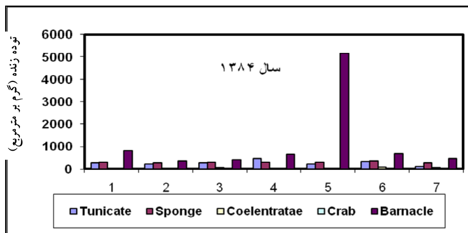
نمودار ۱۰-۲: میزان توده زیاده گروههای اصلی روی انواع سازه در سال ۱۳۸۴
