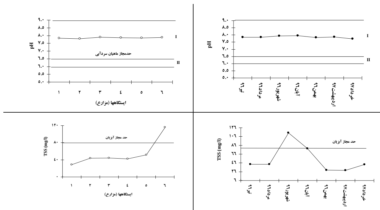
شکل ۴: تغییرات pH و کل مواد جامد معلق در ماهها و ایستگاهها (مزارع پرورش ماهی قزل آلا) به همراه حد مجاز در رودخانه هراز (سال ۱۳۹۶-۹۷)
