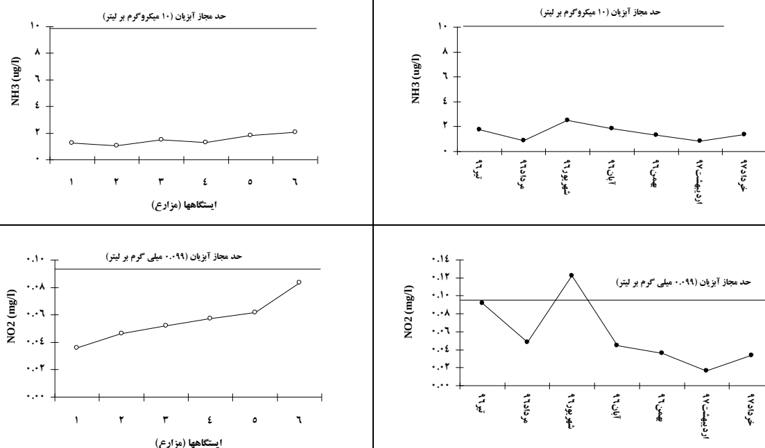
شکل ۶: تغییرات آمونیاک و نیتريت در ماه‌ها و ایستگاه‌ها (مزارع پرورش ماهی قزل آلا) به همراه طبقه بندی در رودخانه هراز (سال ۹۷-۱۳۹۶) Figure 6: \text{NH}_3 and \text{NO}_2 changes of the Haraz River at different months and stations (Rainbow trout farms) (2017-2018).
