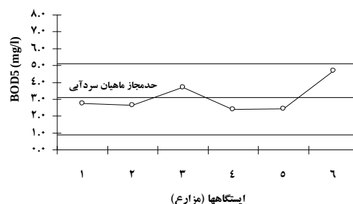
شکل ۳: تغییرات اکسیژن محلول، درصد اشباعیت، اکسیژن خواهی بیولوژیک و شیمیایی در ایستگاه‌ها (مزارع پرورش ماهی قزل آلا) به‌همراه حد مجاز در رودخانه هراز (سال ۹۷-۱۳۹۶)
