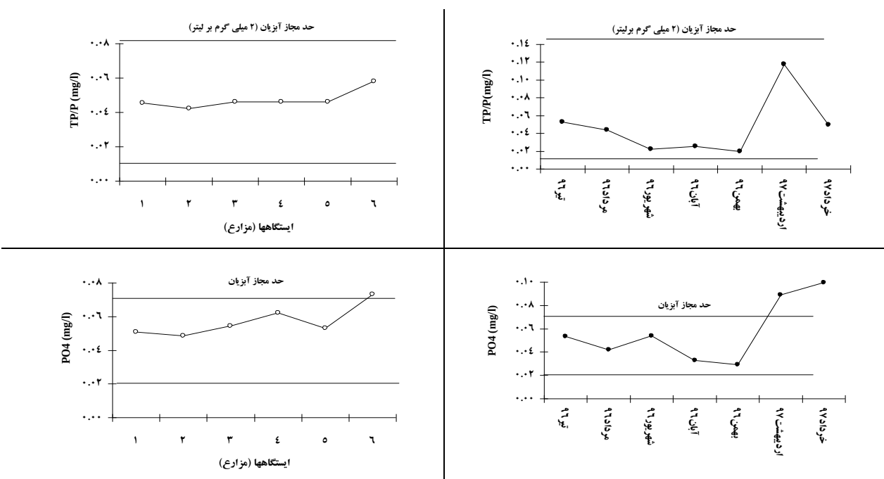
شکل ۵: تغییرات فسفرکل و فسفات در ماهها و ایستگاهها (مزارع پرورش ماهی قزل آلا) به همراه حد مجاز در رودخانه هراز (سال ۱۳۹۶-۹۷)
