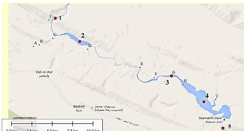
شکل ۱: موقعیت جغرافیایی ایستگاه‌های نمونه برداری دریاچه سد سمیره
