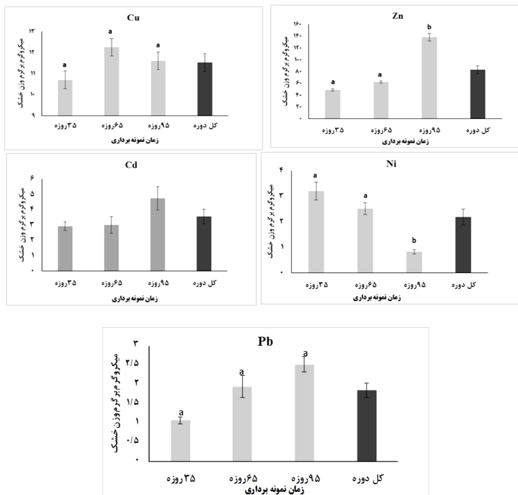
شکل ۱: مقایسه تغییرات میانگین ( \pm انحراف معیار) غلظت فلزات سنگین مس (Cu)، روی (Zn)، کادمیوم (Cd)، نیکل (Ni)، سرب (Pb) در بافت عضله میگوی پرورشی وانامی ( Litopenaeus vannamei ) در سه دوره زمانی و کل دوره ۱۳۹۷. حروف همانم کوچک نشان دهنده عدم اختلاف معنی داری غلظت فلز در بین سه دوره می باشد ( p > 0.05 ).
