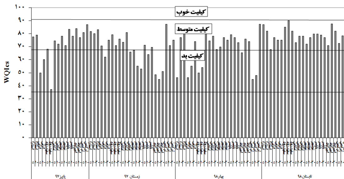
شکل ۳: مقادیر شاخص کیفیت آب در نیم خطها، اعماق و فصول مختلف حوزه جنوبی دریای خزر (۱۳۹۷-۹۸) Figure 3: Water quality index values at different transects, depths and seasons in the southern Caspian Sea basin (2018-2019)
