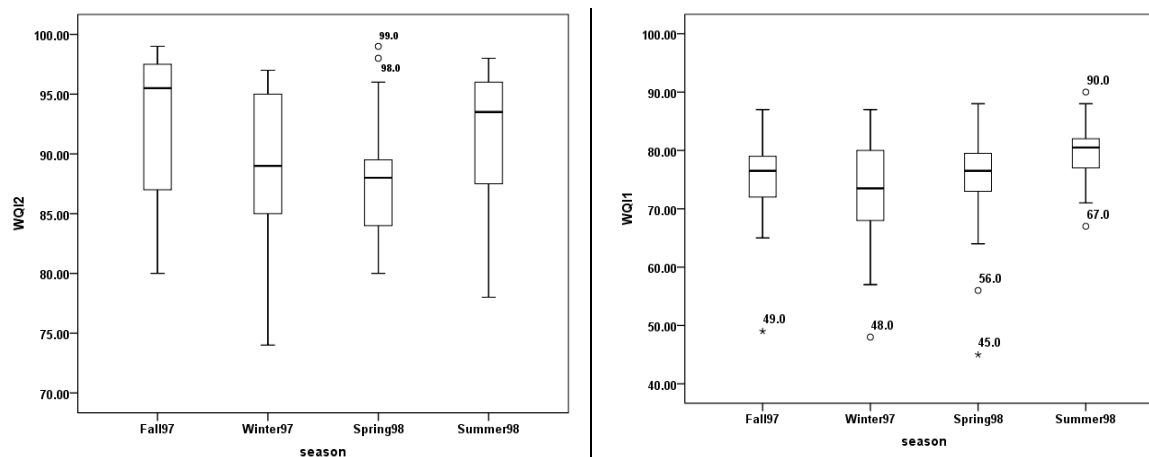
شکل ۴: نمودار جعبه‌ای تغییرات فصلی شاخص کیفیت آب حوزه جنوبی دریای خزر (۱۳۹۷-۹۸) WQI1: پارامترها و وزن‌ها بر اساس مطالعات گذشته نگر (Retrospective studies) دریای خزر: پارامترها و وزن‌ها بر اساس مطالعه Nguyen و همکاران (۲۰۱۳)
