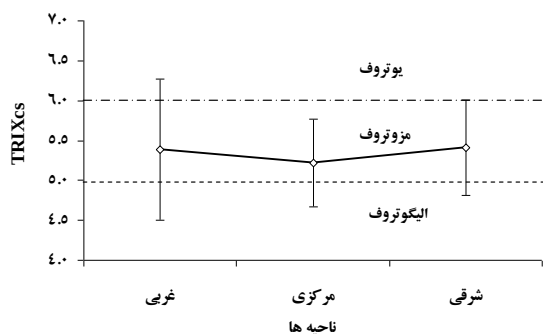
شکل ۲: تغییرات زمانی-مکانی سطح تروفیک TRIXcs و UNTRIX در سواحل ایرانی حوزه جنوبی دریای خزر (۱۳۹۷-۹۸)
