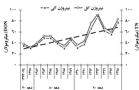
شکل ۶: تغییرات سالانه دراز مدت (۹۸-۱۳۷۳) غلظت فرم‌های مختلف نیتروژن در لایه سطحی حوزه جنوبی دریای خزر
