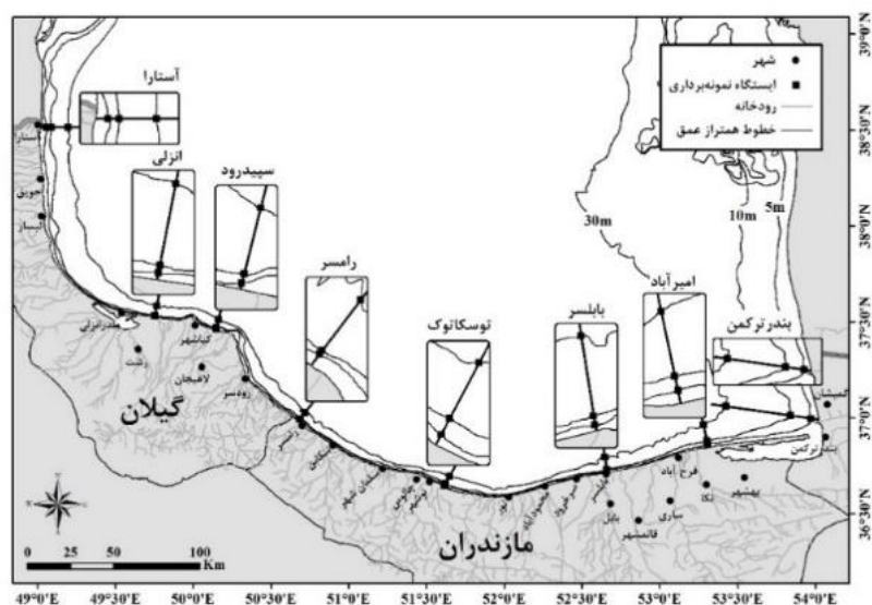
شکل ۱. ایستگاه‌های نمونه‌برداری به همراه نیم خط‌ها و اعماق مختلف در نوار ساحلی حوزه جنوبی دریای خزر (۱۳۹۷-۹۸)
