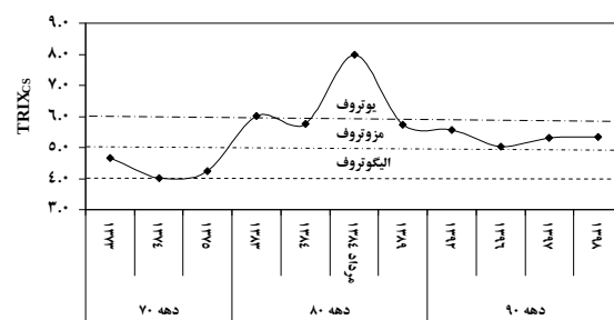
شکل ۸: تغییرات دراز مدت (۹۸-۱۳۷۳) سطح تروفتیک TRIXcs و UNTRIX در سواحل ایرانی حوزه جنوبی دریای خزر (داده‌های مرداد ۱۳۸۴ برگرفته از Soloviev (2005) می‌باشد)
