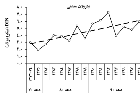
شکل ۶: تغییرات سالانه دراز مدت (۹۸-۱۳۷۳) غلظت فرم‌های مختلف نیتروژن در لایه سطحی حوزه جنوبی دریای خزر
