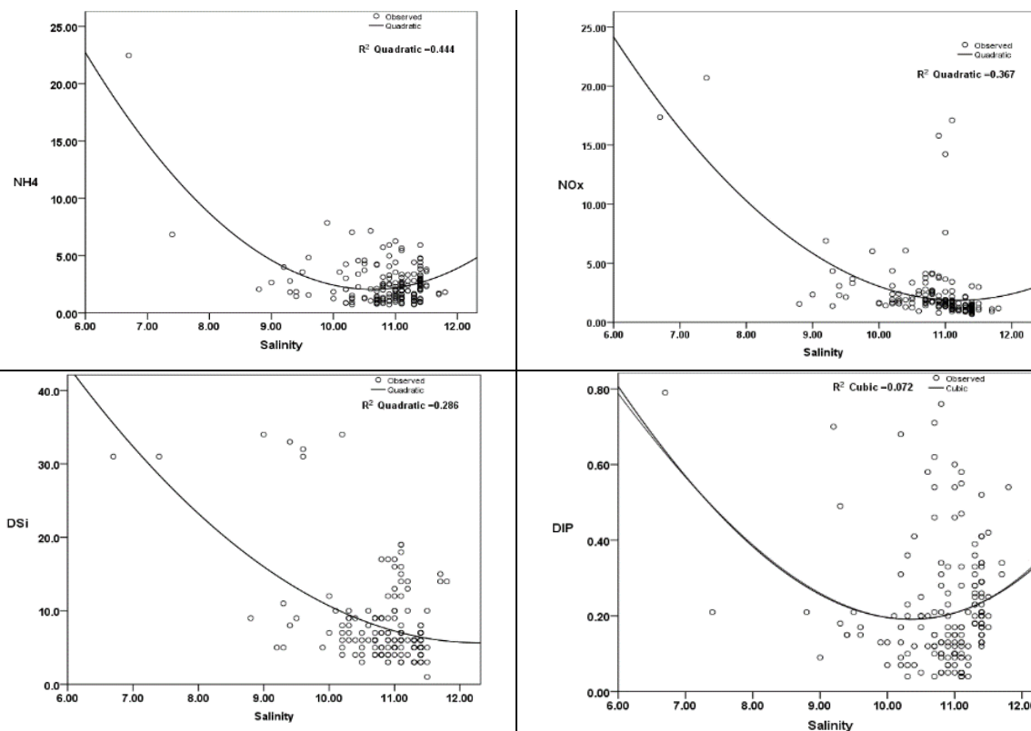
شکل ۵: پراکندگی سالانه غلظت \text{NH}_4 ، \text{NO}_x ، \text{DIP} و \text{DSi} در مقابل شوری در آب‌های ساحلی حوزه جنوبی دریای خزر (۱۳۹۷-۹۸)
