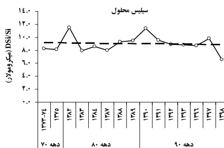
شکل ۷: تغییرات سالانه دراز مدت (۹۸-۱۳۷۳) غلظت فرم‌های مختلف فسفر و سیلیس محلول در لایه سطحی حوزه جنوبی دریای خزر
