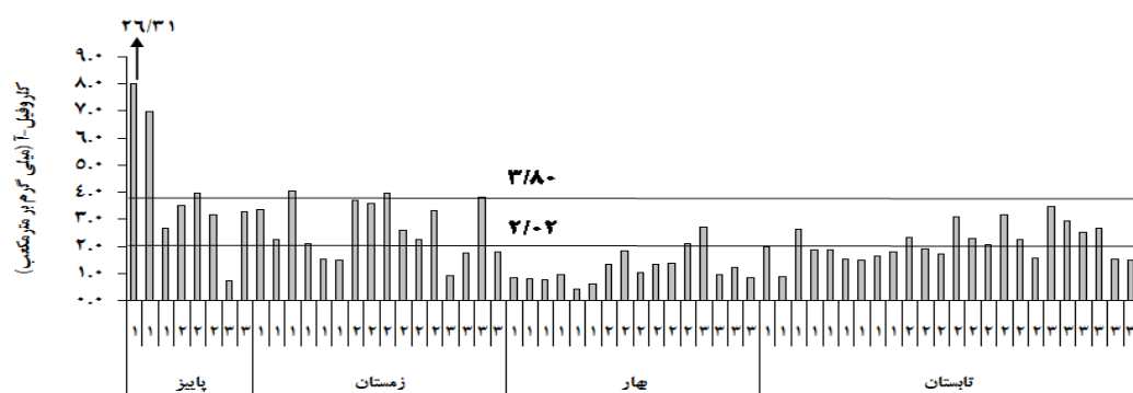
شکل ۲: تغییرات غلظت کلروفیل در فصول و نواحی مختلف در سواحل ایرانی دریای خزر (۱۳۹۷-۹۸)
