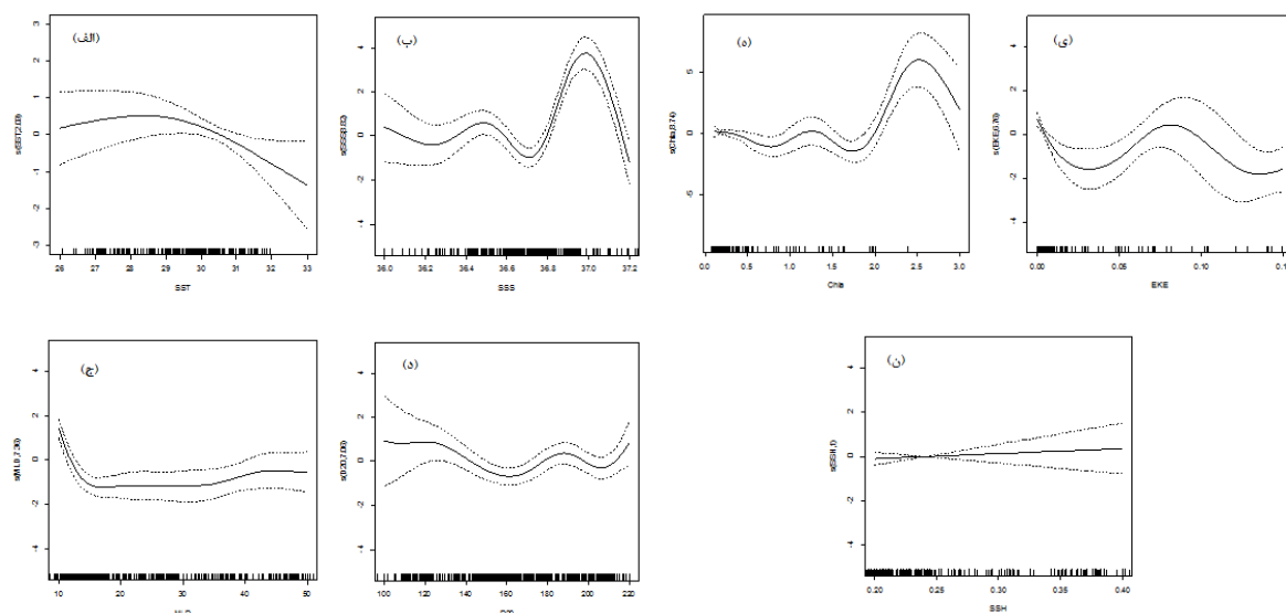
شکل ۴: نمودار تاثیر مدل در متغیرهای محیطی از جمله (الف) دمای سطحی آب دریا، (ب) شوری سطحی آب دریا، (ج) عمق لایه مخلوط شونده، (د) عمق هم‌دمای ۲۰ درجه سانتی گراد، (ه) کلروفیل آ سطحی آب دریا، (ی) انرژی جنبشی ادی و (ن) ارتفاع سطح آب دریا در ارتباط با میزان صید به ازاء واحد تلاش (CPUE) تون هوور معمولی. خط تیره بیانگر معادله مناسب مدل (fitted GAM function) و خط نقطه‌چین بیانگر فاصله اطمینان ۹۵٪ (95% confidence intervals) می‌باشد.
