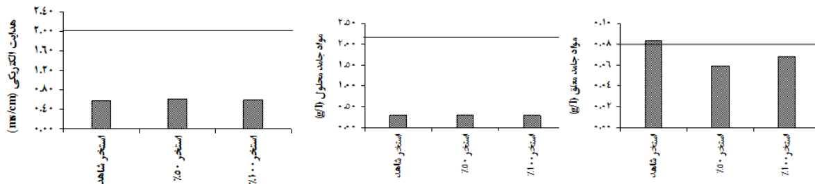
شکل ۴: تغییرات هدایت الکتریکی، مواد جامد محلول و معلق آب به همراه استانداردهای پرورش قزل آلا در استخرهای مختلف
