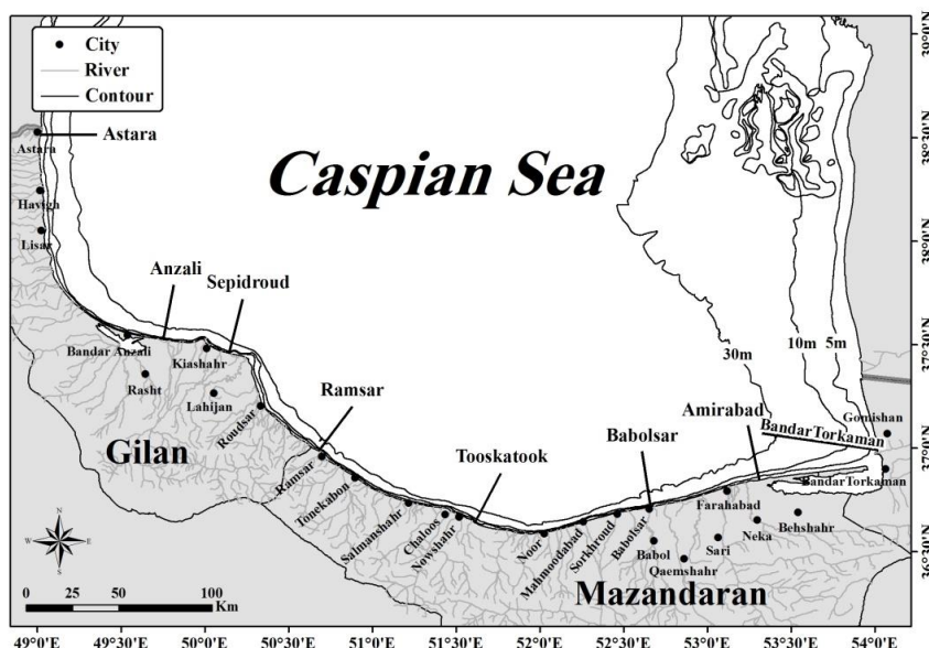
شکل ۱: موقعیت ایستگاه‌ها و نیمه‌های نمونه‌برداری در حوزه جنوبی دریای خزر Figure 1: Location of sampling stations and transects in the southern basin of Caspian Sea
