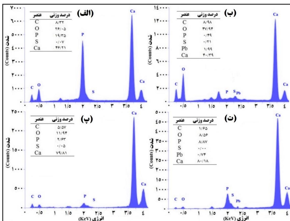
شکل ۴: طیف‌های EDX مربوط به متغیرهای پاسخ PbR: (الف) قبل از جذب زیستی سرب، (ب) بعد از جذب زیستی سرب) و PbO (پ: قبل از جذب زیستی سرب، ت: بعد از جذب زیستی سرب). جداول داخل شکل: ترکیب عنصری جاذب‌ها (درصد وزنی)
