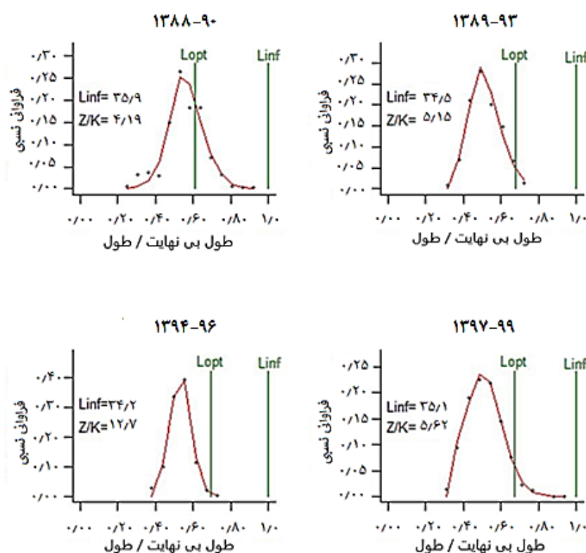
شکل ۱: نتایج آنالیز مدل LBB برای گونه ماهی کلمه خزری در سواحل جنوب شرقی دریای خزر در ۴ دوره زمانی مختلف (۱۳۸۸-۹۹) Figure 1: The result of LBB model analyse for Caspian Roach species in the southeast coast of the Caspian Sea in 4 different time periods (2009-2020)
