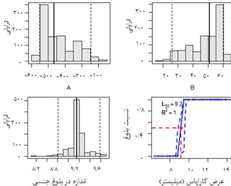
شکل ۱۲: برآورد اندازه طول بلوغ جنسی ( CW_{50} ) جنس ماده خرچنگ Austruca iranica به روش بیزی Figure 12: Estimating of sexual maturity length ( CW_{50} ) in female crab of Austruca iranica by Bayesian method
