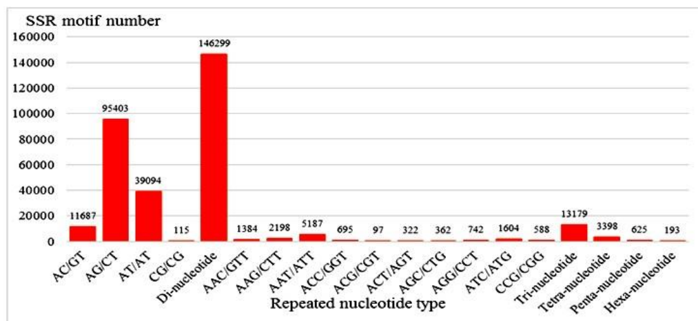
شکل ۳: توزیع فراوانی توالی‌های کوتاه تکراری (SSR) بر پایه نوع موتیف
