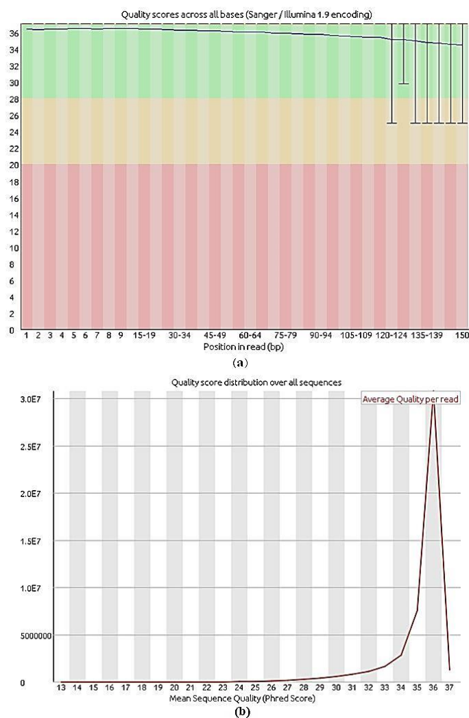
شکل ۲: نمودار کیفیت توالی‌یابی به ازای هر باز (a) و امتیاز کیفیت به ازای توالی (b) Figure 2. Quality assessment tests. (a) per base and (b) per sequence quality scores
