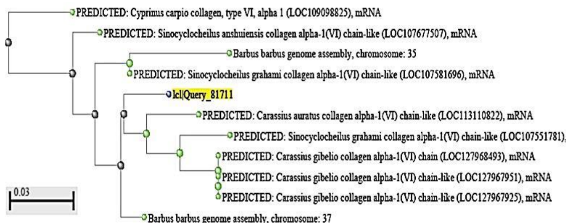
شکل ۴: رابطه فیلوژنتیک جایگاه MN1359 با سایر توالی‌های موجود در پایگاه داده NCBI
