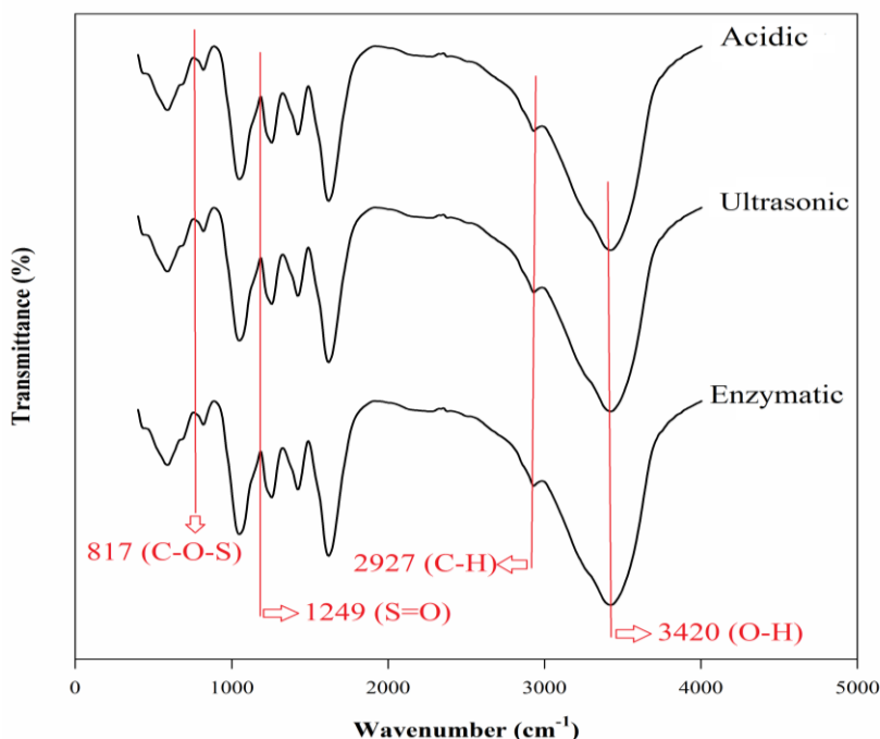
شکل ۲: طیف FTIR فوکوئیدان‌های استخراج شده از جلبک Sargassum ilicifolium به روش‌های مختلف Figure 2: FTIR spectra of fucoidan extracted from Sargassum ilicifolium by different methods
