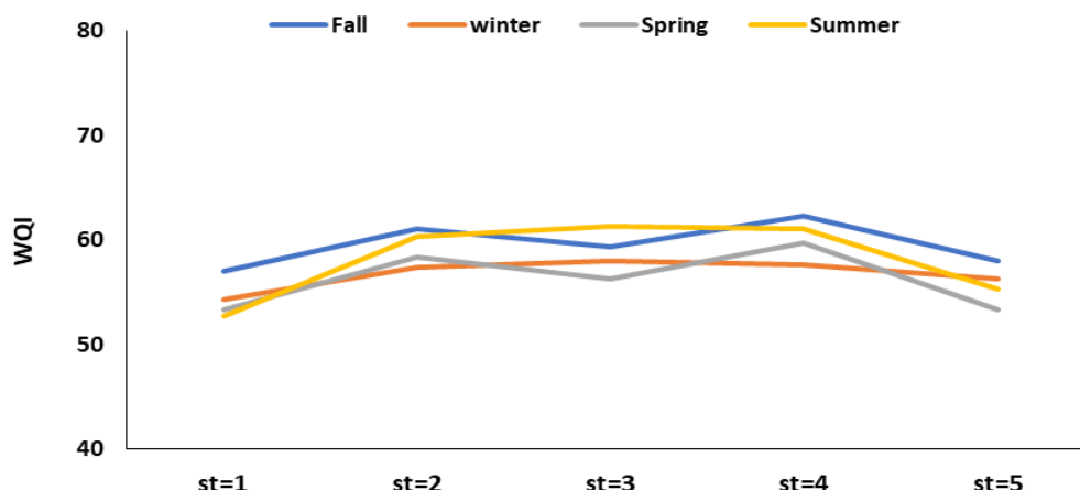
شکل ۱: مقدار شاخص WQI در ایستگاه‌های مورد مطالعه فصول مختلف در دریاچه پشت سد مارون (۱۳۹۹-۱۴۰۰)
