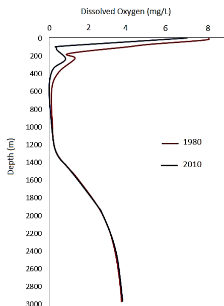
شکل ۶: مقایسه پروفیل میانگین سالانه اکسیژن محلول دریای
