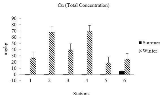
شکل ۳: مقایسه تغییرات میانگین غلظت کل فلز مس (میلی گرم بر کیلوگرم) ± خطای استاندارد میانگین در رسوبات ایستگاه‌های مختلف رودخانه سیروان در فصل‌های تابستان و زمستان ۱۴۰۲
