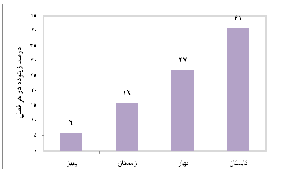
نمودار ۲: نسبت زیتوده جلبکهای قرمز نمونه‌برداری شده در هر فصل (درصد زیتوده در سال)
