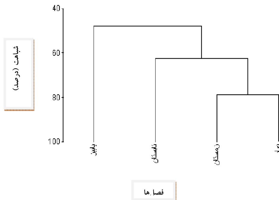
نمودار ۴: مقایسه شبهات فصول مختلف نمونه برداری از نظر مقدار زیتوده جلبکهای قرمز
