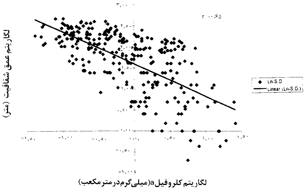
نمودار ۲: همبستگی بین لگاریتم عمق شفافیت و لگاریتم کرو فیل a در حوضه جنوبی دریای خزر (سال ۱۳۷۵)
