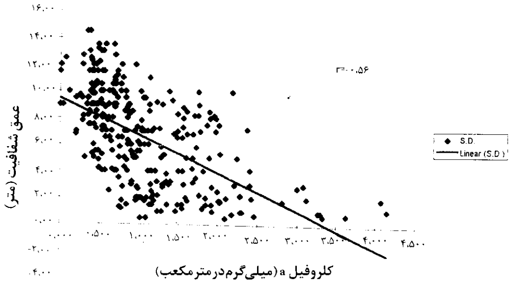
نمودار ۱: همبستگی بین عمق شفافیت و کرو فیل a در حوضه جنوبی دریای خزر (سال ۱۳۷۵)
