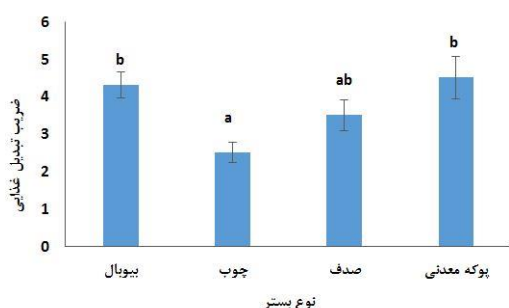
شکل ۳: مقایسه ضریب تبدیل غذایی ماهیان پرورش یافته در سیستم مدار بسته طراحی شده با بسترهای متفاوت
