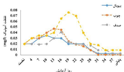
شکل ۲: میانگین سطح آمونیاک اندازه گیری شده در آکواریوم‌های دارای بسترهای مختلف در یک دوره ۴۰ روزه
