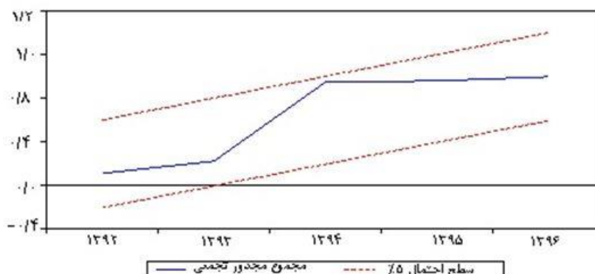
شکل ۱: نتایج آزمون ثبات ضرایب مجموع مجذور تجمعی (CUSUMSQ) Figure 1: Results of CUSUMSQ coefficients stability test.
