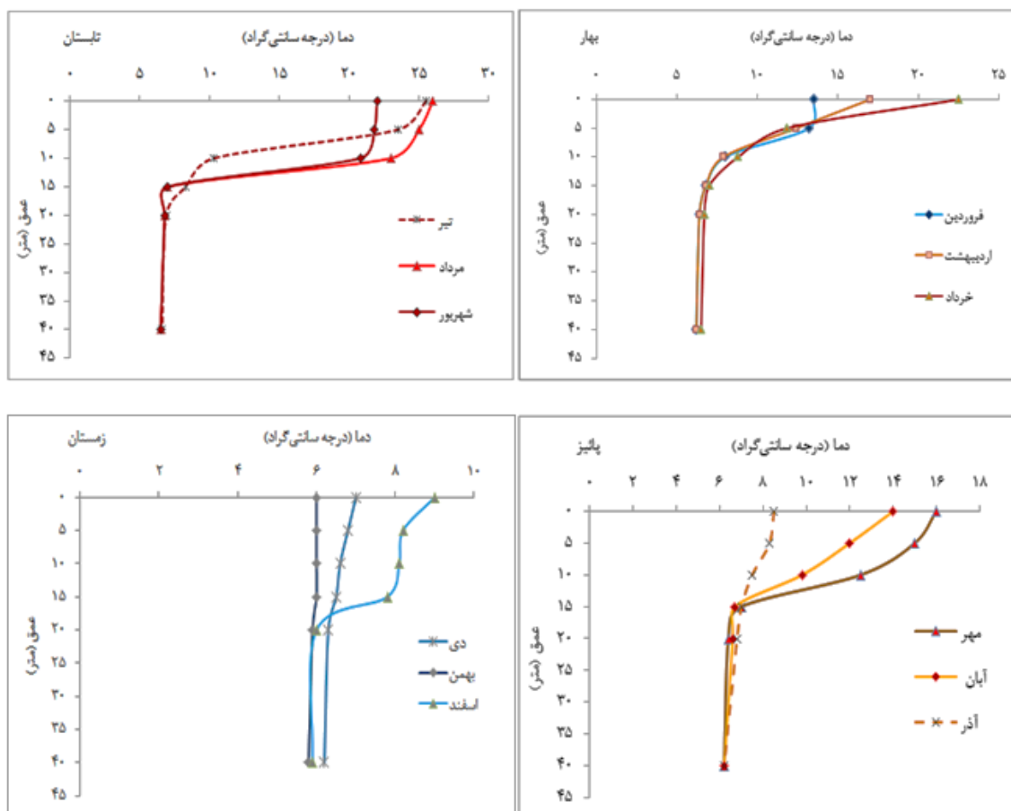
شکل ۲: تشکیل و از بین رفتن لایه‌بندی دمایی طی فصول مختلف در دریاچه سد گاران ، ۱۳۹۶-۱۳۹۷ Figure 2: Formation and vanishing of thermal stratification during different seasons at Marivan Garan dam (2017-2018)
