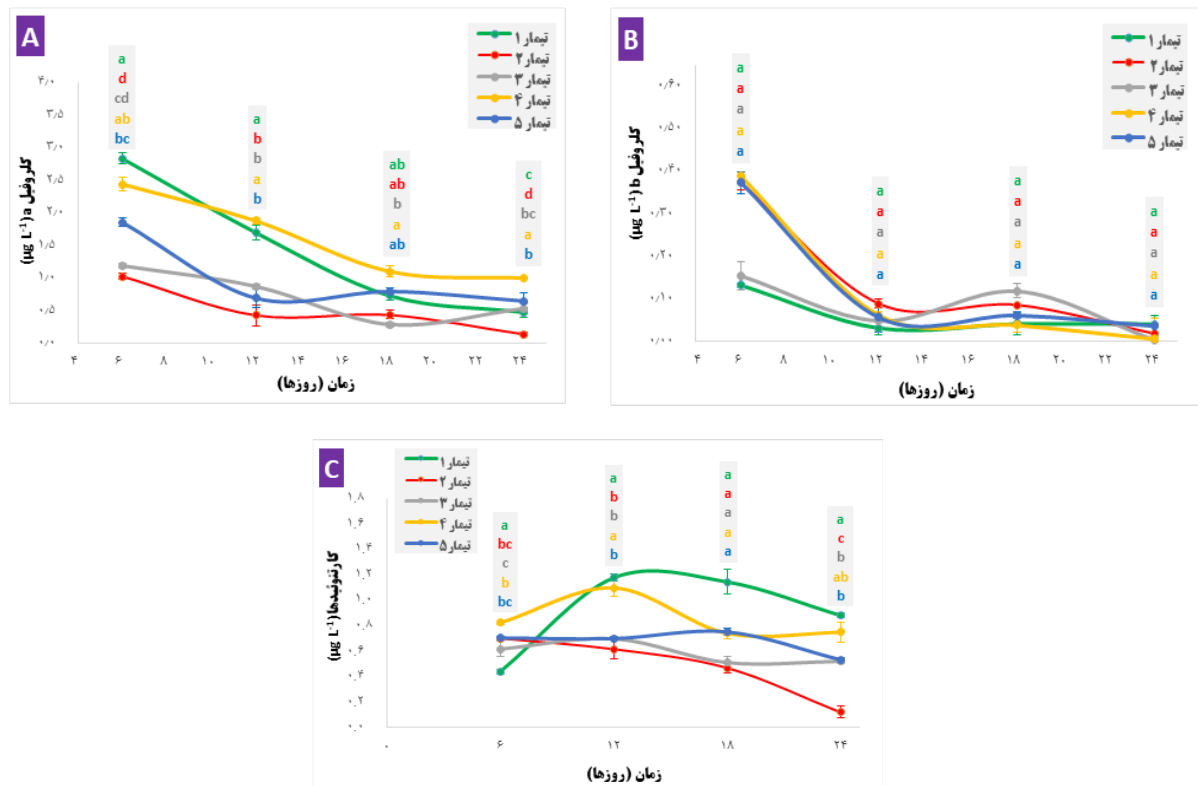
شکل ۵: مقایسه میزان رنگیزه‌های فتوسنتزی: کلروفیل a (A)، کلروفیل b (B) و کارنوئیدها (C) جلبک D. salina در تیمارهای مختلف در طول دوره ۲۴ روزه
