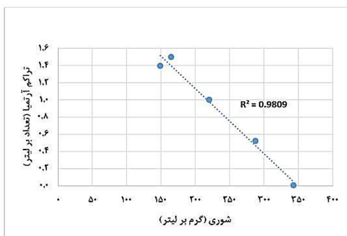
شکل ۳: منحنی همبستگی بین میزان شوری آب دریاچه ارومیه و تراکم آرتمیا (زمانی که تراکم آرتمیا را در سطر سوم جدول ۱ (سال ۱۳۵۶، به جای ۳ عدد در لیتر، ۱ عدد در لیتر در نظر گرفته شده است).
